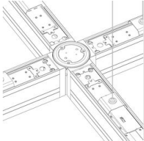
2029 Joint circulaire X
