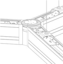
2028 Joint en Y circulaire
