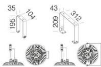
Support mural réglable
