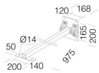
42 Bras orientable
