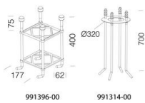
299 Tirefonds
