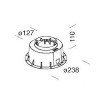
313 Boîte d'encastrement
