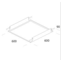
Telaio - 600x600
