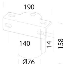
236 Fijación columna 76mm
