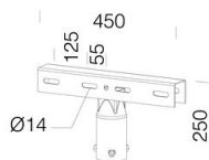
59 Soporte para columna
