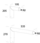
205 Fijación cabeza-columna
