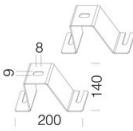
39 Fijación en plafón
