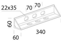
345 Soporte a pared
