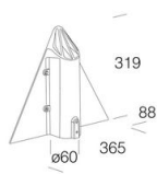
96 Fijación a columna ø60 - Meridiana
