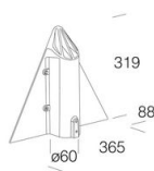
96 Fijación a columna ø60 - Meridiana
