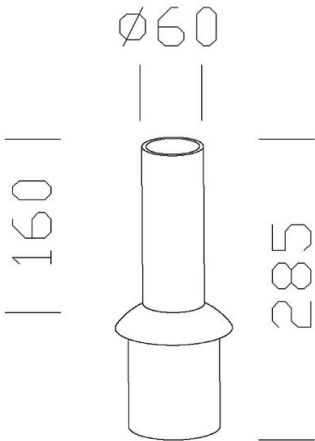
528 Racor cabeza-columna 60mm
