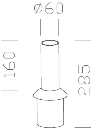
528 Racor cabeza-columna 60mm
